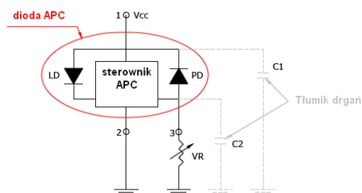
sterownik APC wewnątrz obudowy diody:
