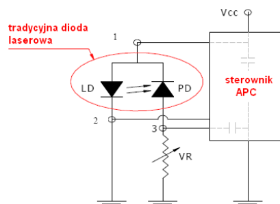
sterownik APC wewnątrz obudowy diody:
