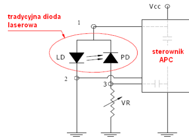
sterownik APC wewnątrz obudowy diody:
